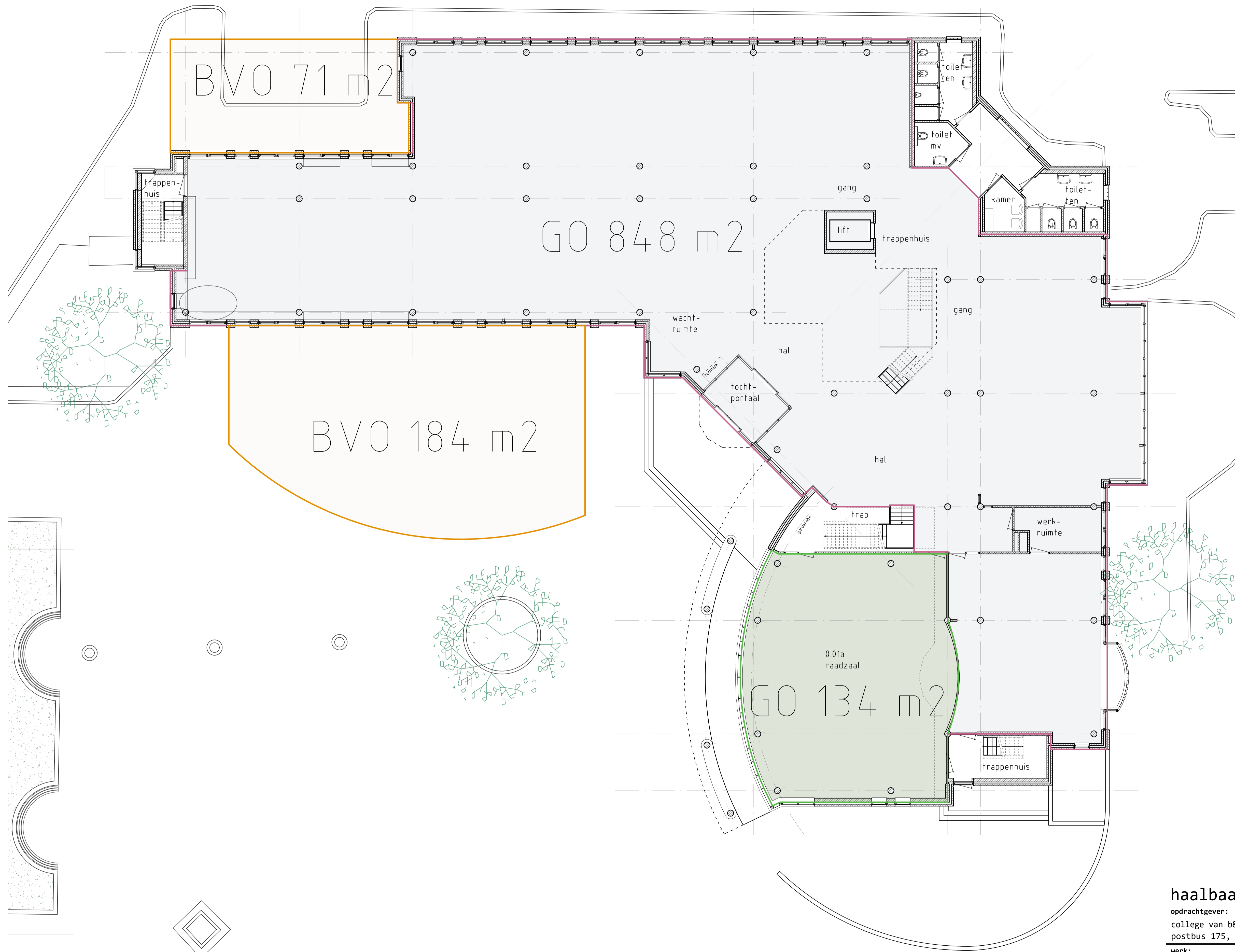
begane grond overzicht oppervlakten
