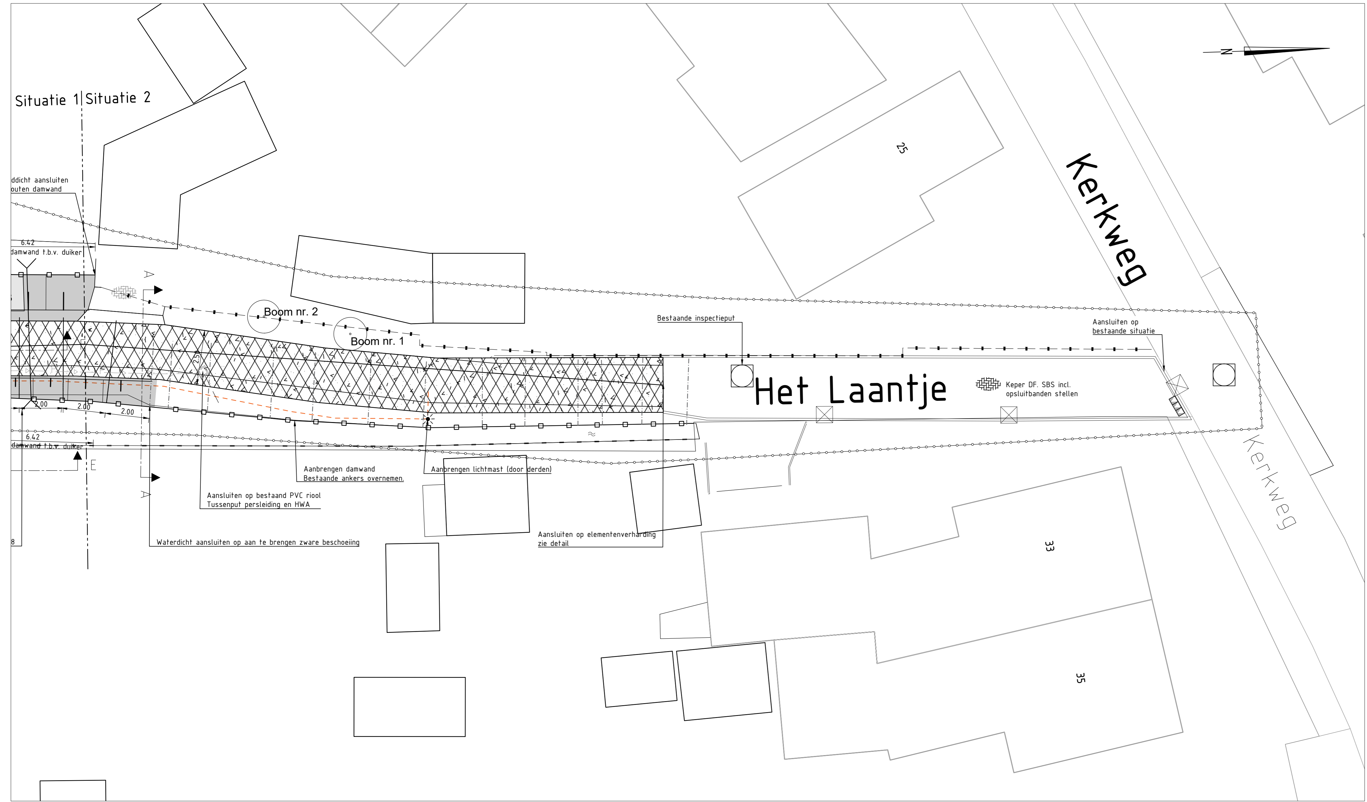
SITUATIE 2 Schaal 1:100
