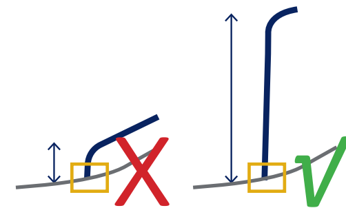
Geen bocht vlak voor het sifon
