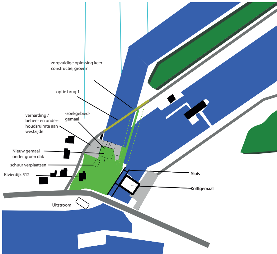
Mogelijke inrichting
