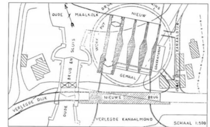
Schets van het nieuwe Lingegemaal te Steenenhoek getekend over de oude situatie heen
